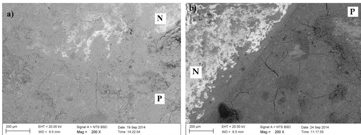
Rys. 5. Przykładowe widoki płaszczyzn zespolenia z wykorzystaniem betonu BR dojrzewającego pod ciśnieniem 0,3 MPa: a) podkład po piaskowaniu, b) podkład kuty; N – materiał naprawczy, P – podkład betonowy
