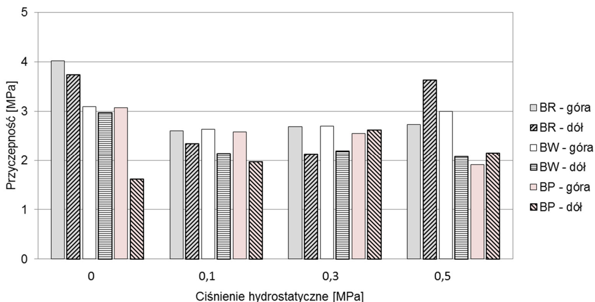
Rys. 3. Przyczepność betonów naprawczych do podkładów pionowych
