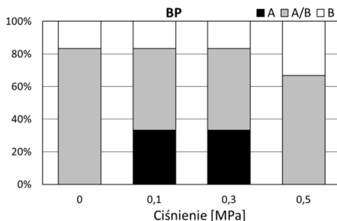
Rys. 4. Procentowy udział typów zniszczeń uzyskany w badaniach przyczepności metodą pull-off: A – zniszczenie kohezyjne w podłożu betonowym, A/B – zniszczenie adhezyjne na powierzchni rozdziálu pomiędzy podkładem a materiałem naprawczym, B – zniszczenie kohezyjne w warstwie naprawczej
