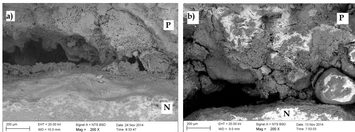
Rys. 6. Wady płaszczyzny zespolenia uzyskane dla betonów naprawczych BP z kopolimerem (ciśnienie 0,5 MPa): pustka powietrzna w płaszczyźnie zespolenia: zaczyn-podkład betonowy, b) widoczne luźne fragmenty podkładu niepowiązane z zaczynem; N – materiał naprawczy, P – podkład betonowy
