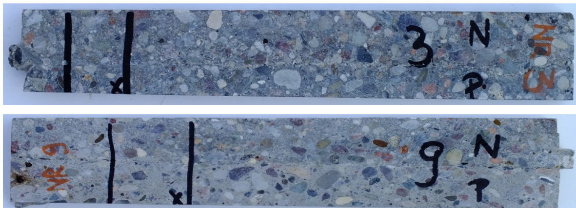
Rys. 2. Przekrój przez warstwę stykową pomiędzy betonem naprawczym (N) a podkładem (P). Czarnymi liniami zaznaczono miejsce pobrania próbki do analizy SEM powierzchni zespolenia. Zdjęcie górne – próbka pobrana z betonu BR (ciśnienie 0,5 MPa), zdjęcie dolne – próbka pobrana z betonu BP (ciśnienie 0,5 MPa)
