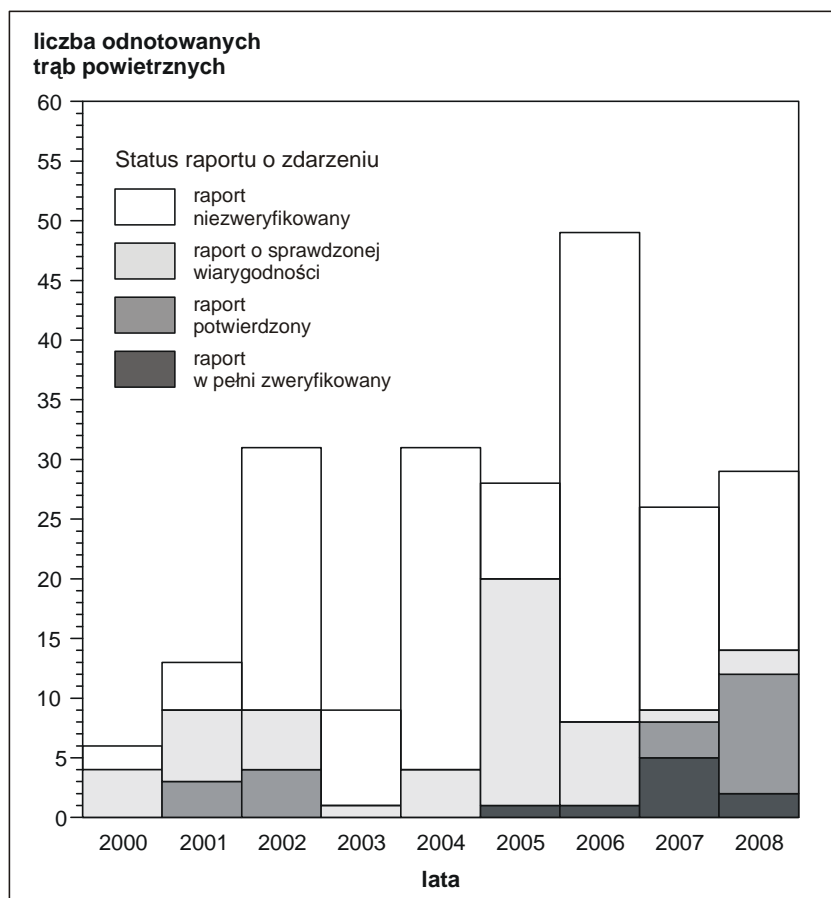
Rys. 3. Liczba odnotowanych trąb powietrznych w Polsce w latach 2000–2008
