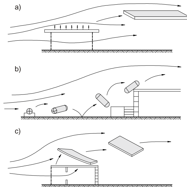
Rys. 5. „Pociski powietrzne” powstające w wyniku: a) sił aerodynamicznych, b) toczenia się i koziołkowania, c) ciśnienia wewnętrznego i zewnętrznego (rozerwania budynku) [8]
