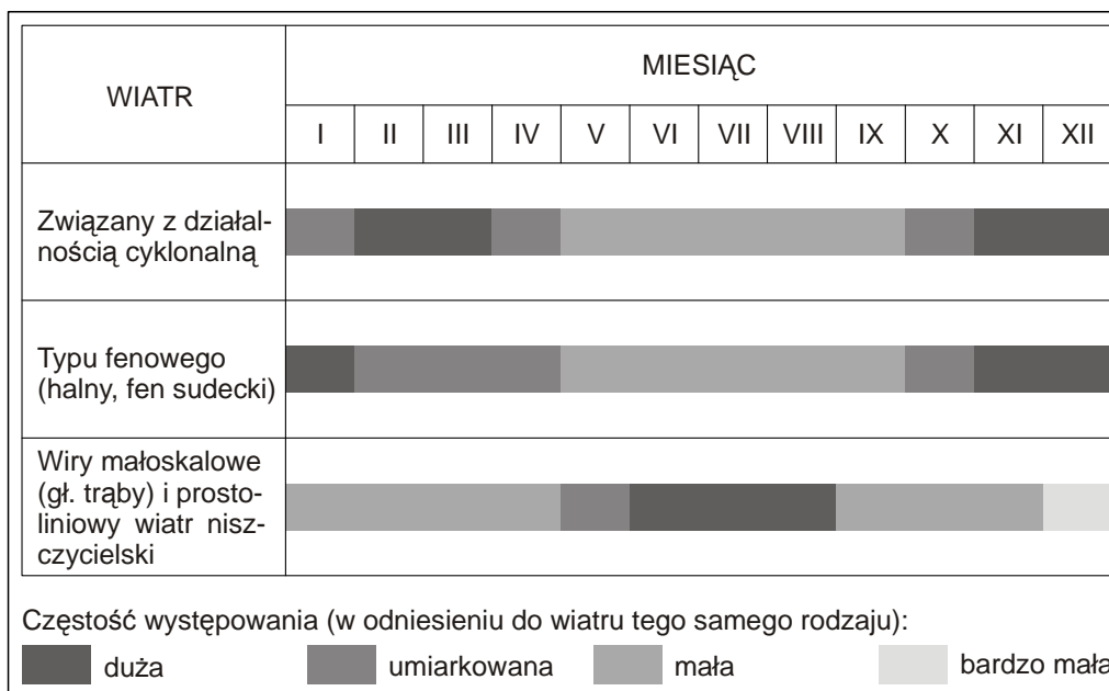
Rys. 2. Okresy występowania w Polsce wiatrów katastrofalnych w zależności od genezy ich powstania (dane dotyczące wiatru związanego z działalnością cyklonalną i wiatru fenowego wg [7])
