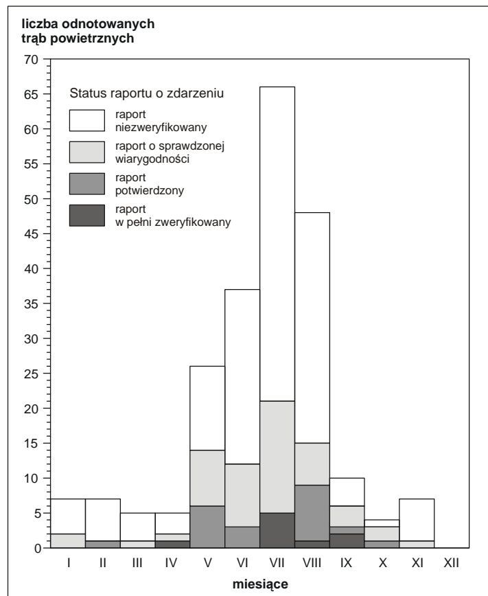
Rys. 4. Miesięczny rozkład występowania trąb powietrznych w Polsce w latach 2000–2008
